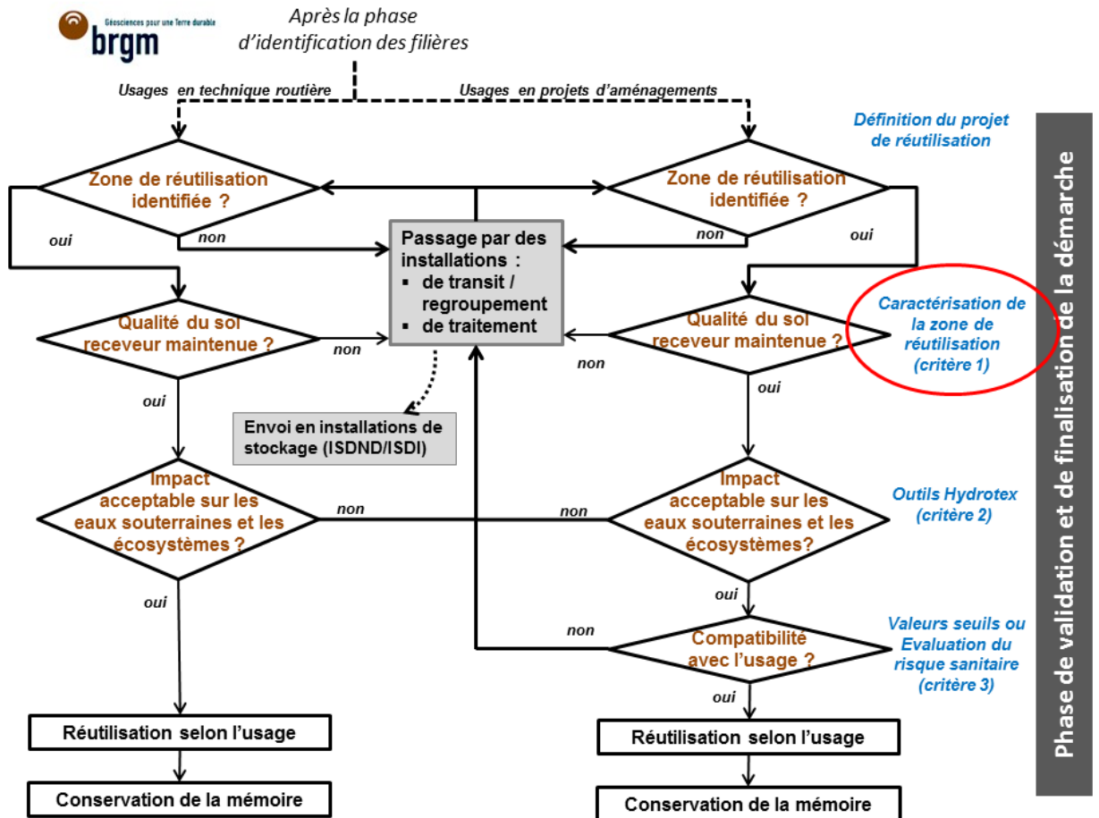
Figure 2 : Schéma des principes de réutilisation hors site des terres excavées (guide BRGM RP-60013)
